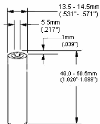
Dimensiones según estándares de ANSI / IEC
