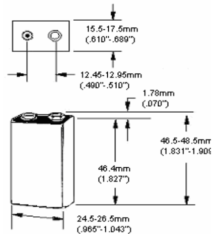
Dimensiones según estándares de ANSI / IEC
